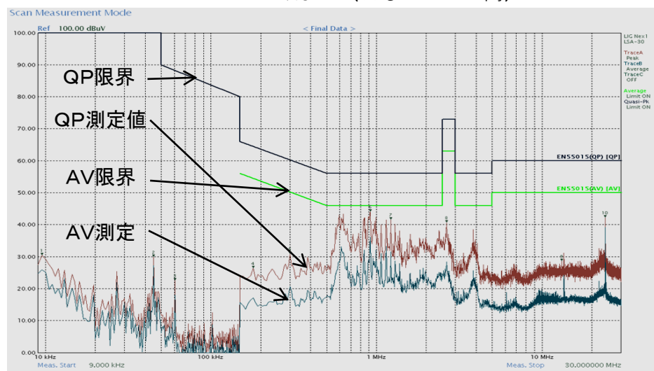
CM Noise (A C とアース間)
